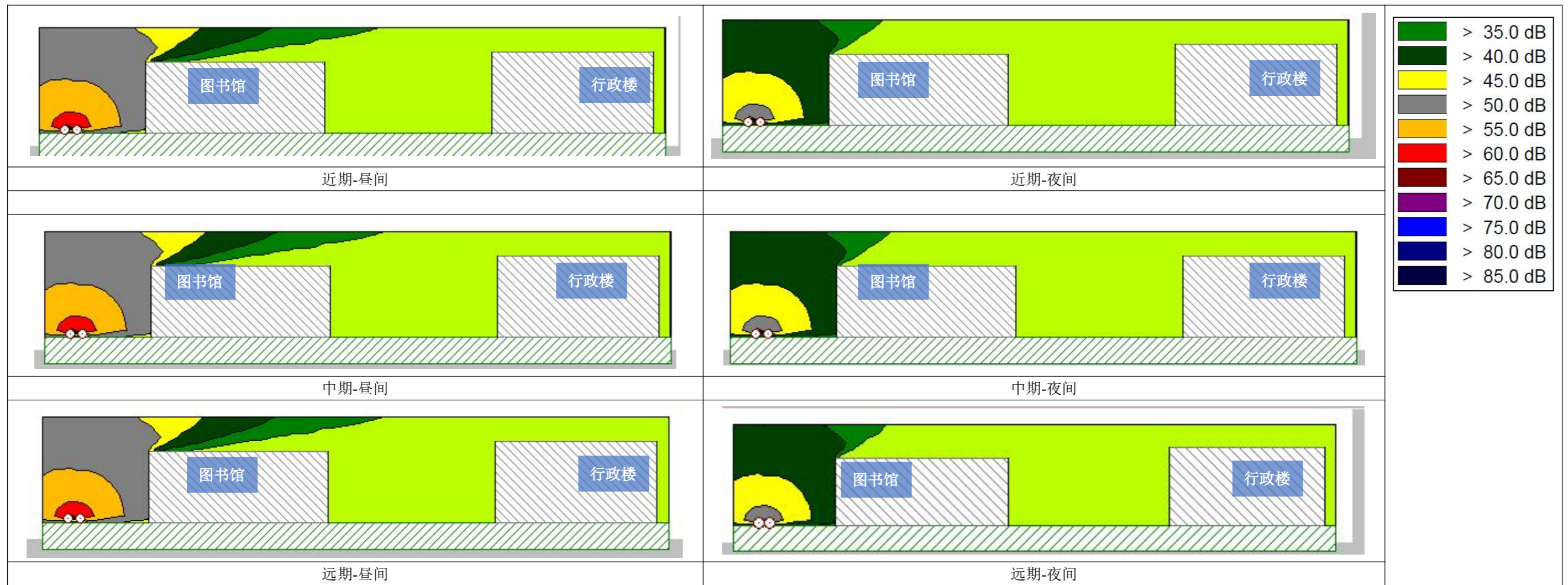
图 5-7 典型敏感点声环境质量预测剖面图
