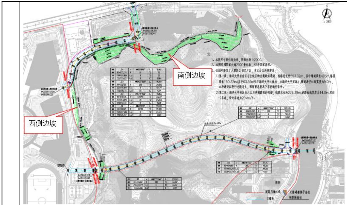
图 2-9 公园环路边坡平面图
