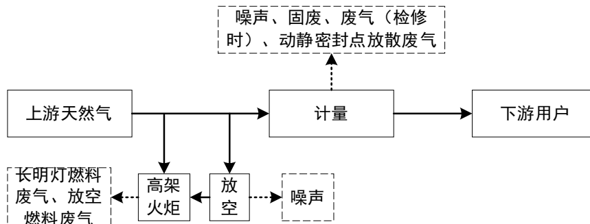
图 2-2 首站污染工艺流程及产污环节图
