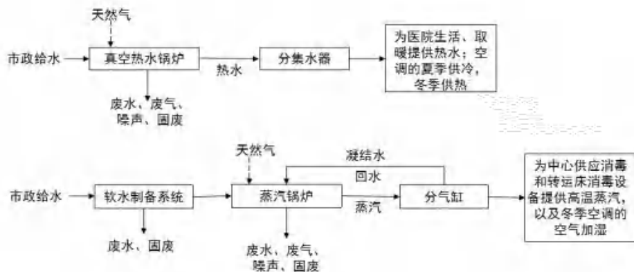
图 2-3 项目主要生产工艺流程图
