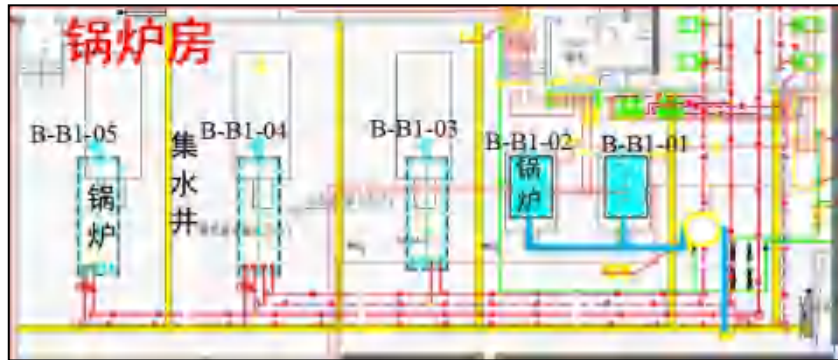
图2-1 锅炉房平面布置图
