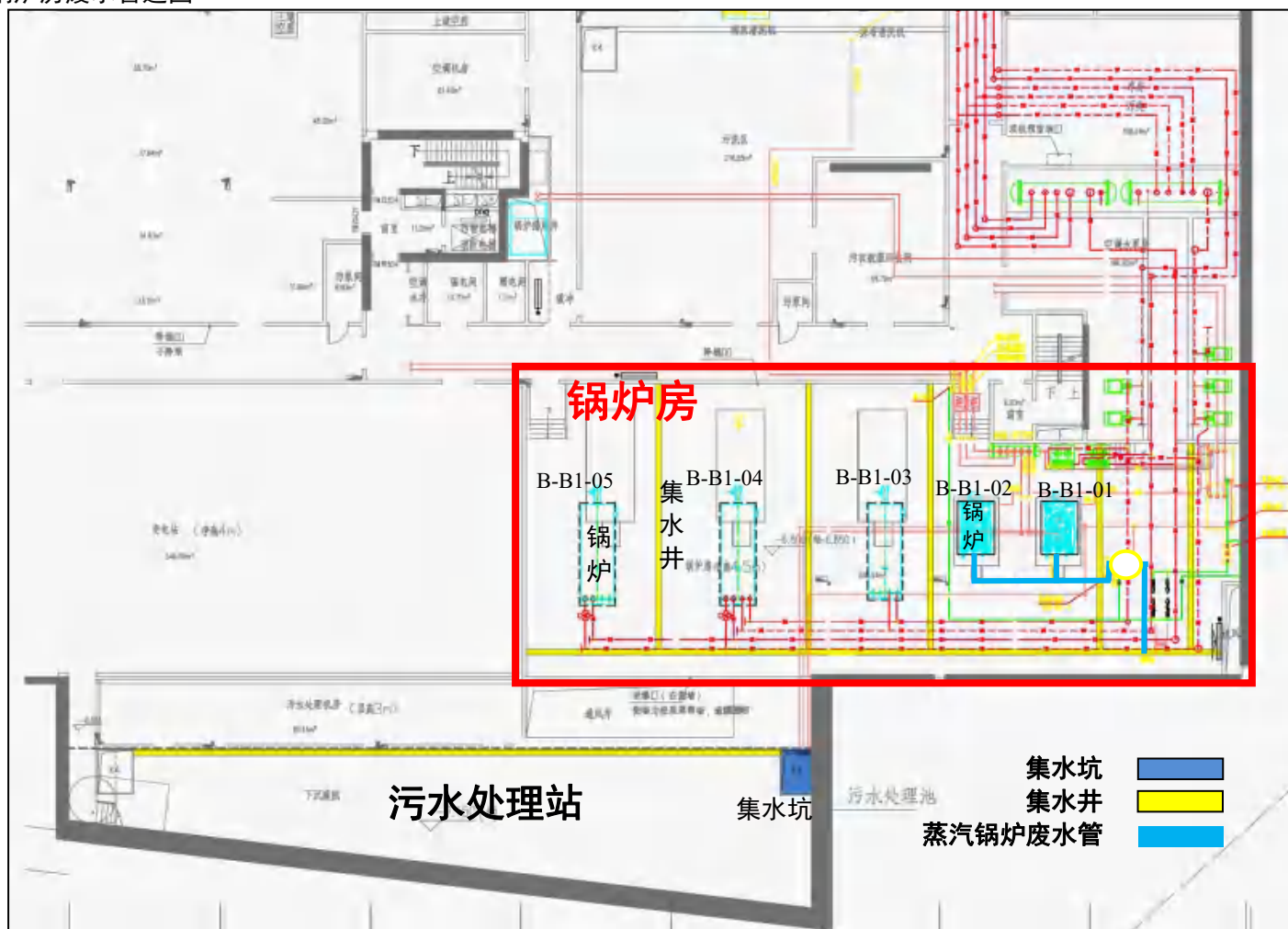
附图 14 项目锅炉房废水管道图
