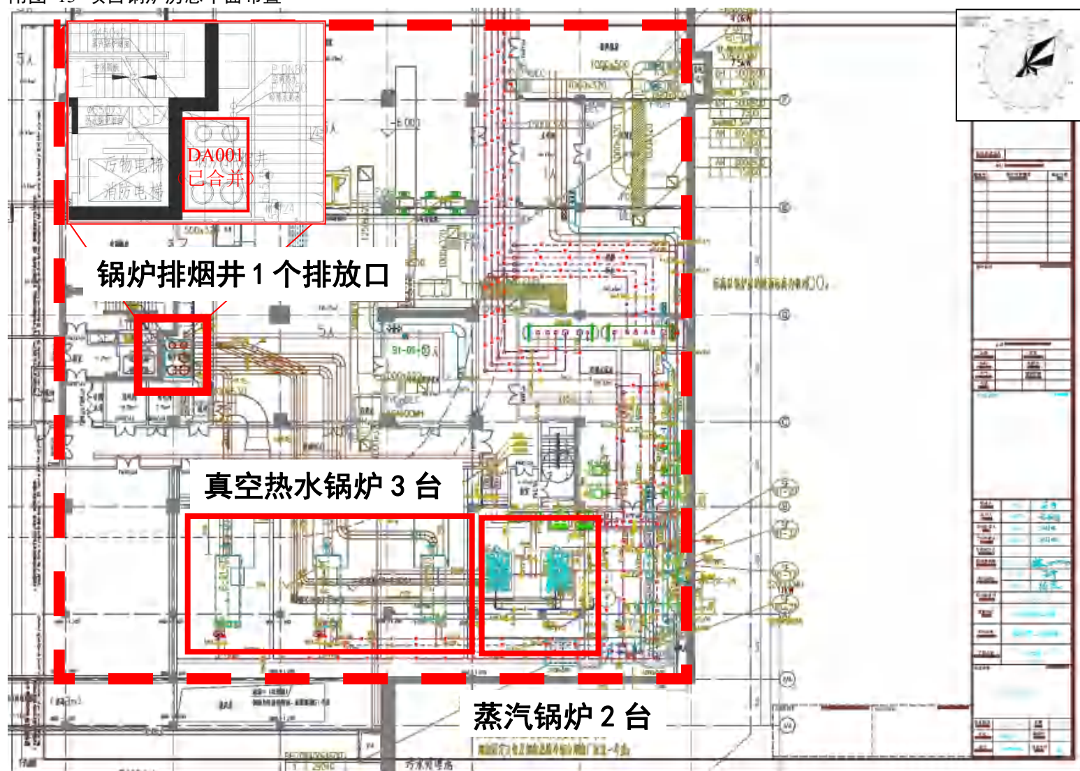
附图 13 项目锅炉房总平面布置
