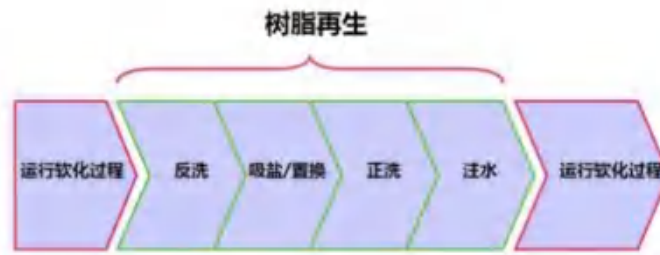
图 2-4 项目软化水工艺流程
