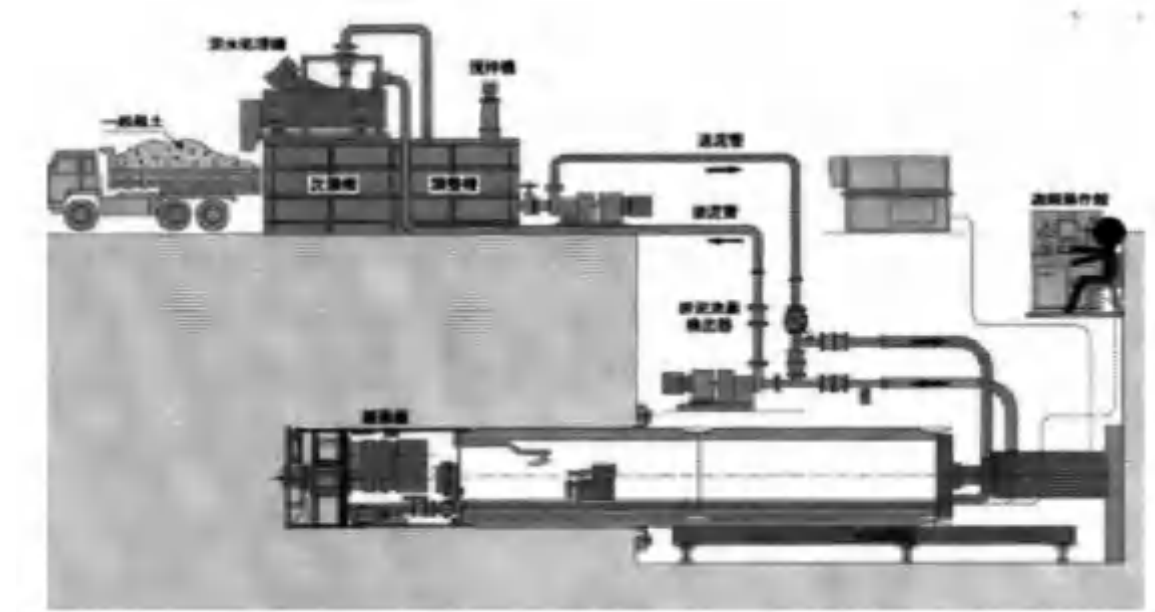
图 4.1-12 顶管穿越示意
