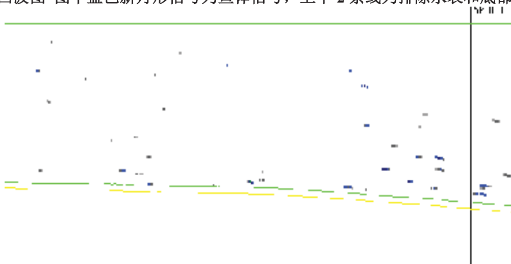
图 5.5-2 单体回波图（此图为上图经处理后排除掉噪声的回波图，剩余的几乎都是鱼体回波信号）
