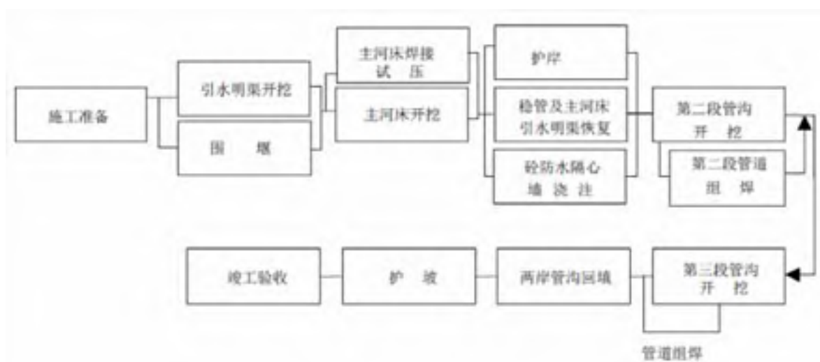
图 4.1-10 导流明渠穿越河流施工流程
