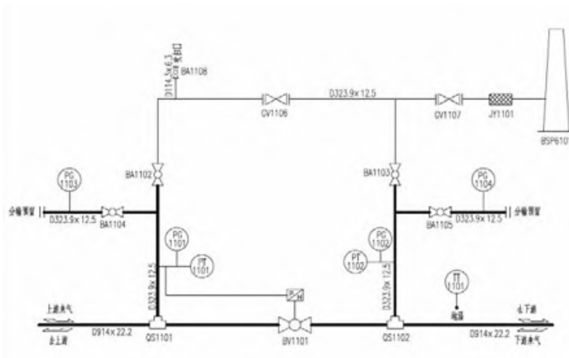
图 3.4-8 典型阀室流程示意图
