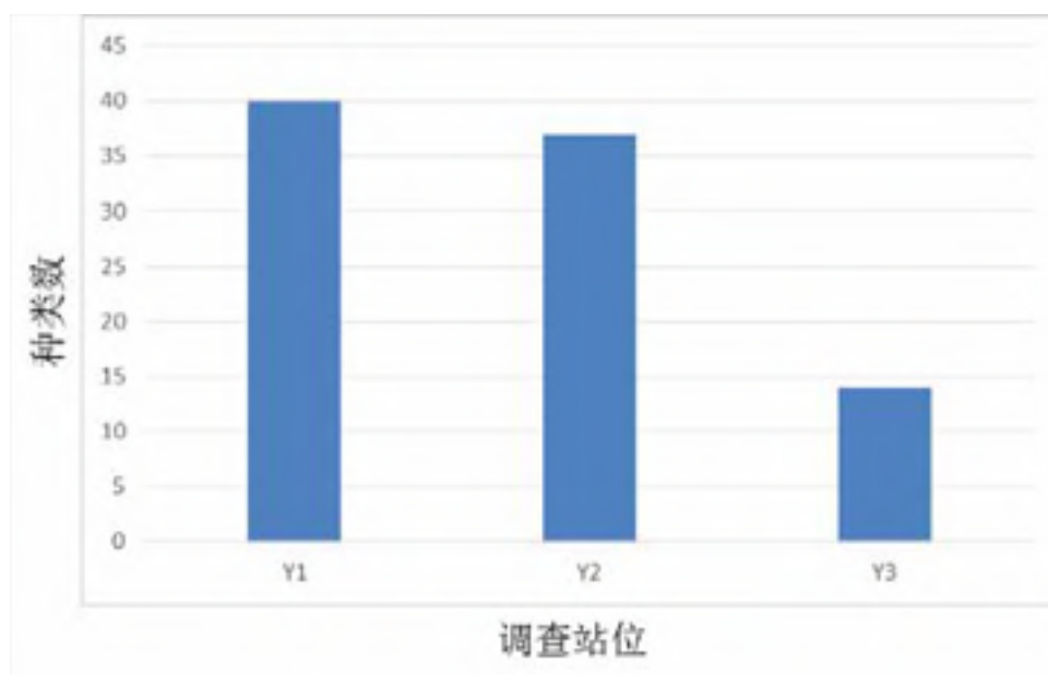
图 5.5-5 调查水域浮游植物种类数空间分布
