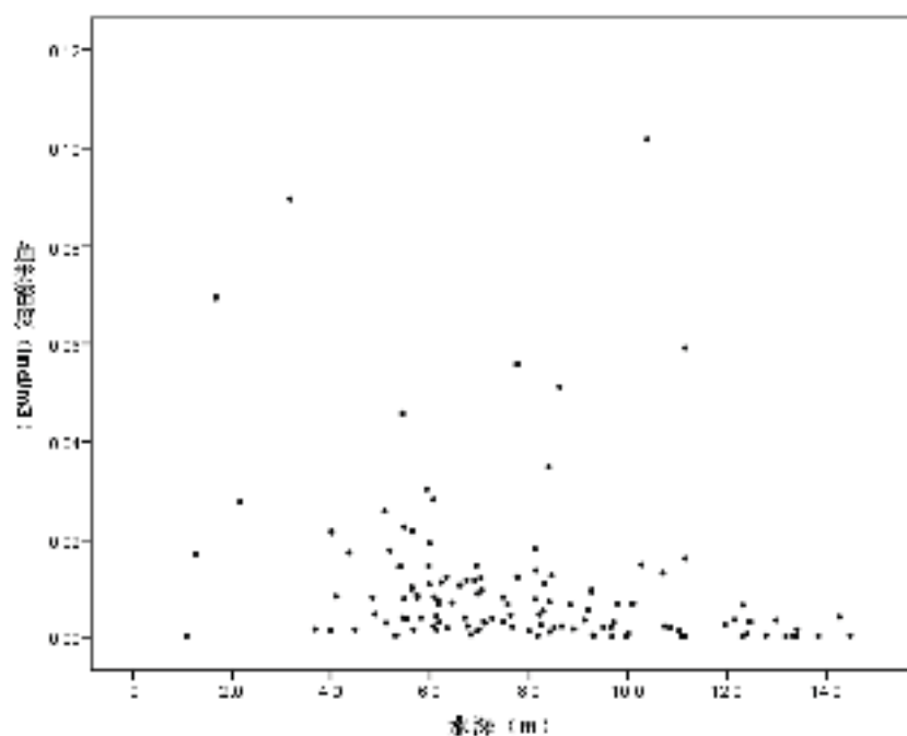
图 5.5-3 2019 年 4 月月份鱼类垂直分布图
