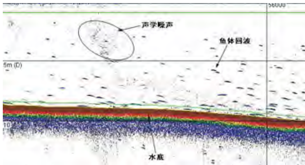
TS 回波图 图中蓝色新月形信号为鱼体信号，上下 2 条线为排除水表和底部噪声
