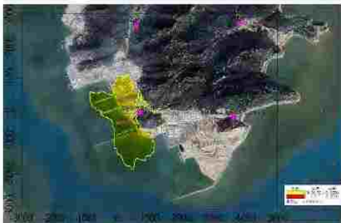
图 8.2-14 1B+3#泊位靠船时 NO 2 叠加现状浓度后 98% 保证率日均质量浓度分布图(µg/m 3 )
