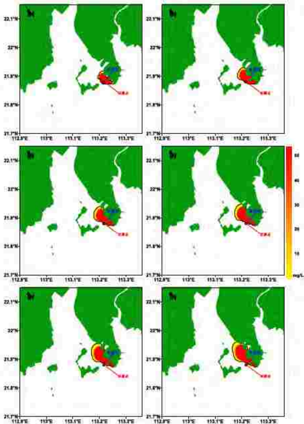
图9.3-19 冬季主导风涨潮时码头前沿操作性泄漏事故硫酸漂移扩散预测结果 (从上至下、左至右为第1至第6小时; 包络线浓度为0.20ug/L)
