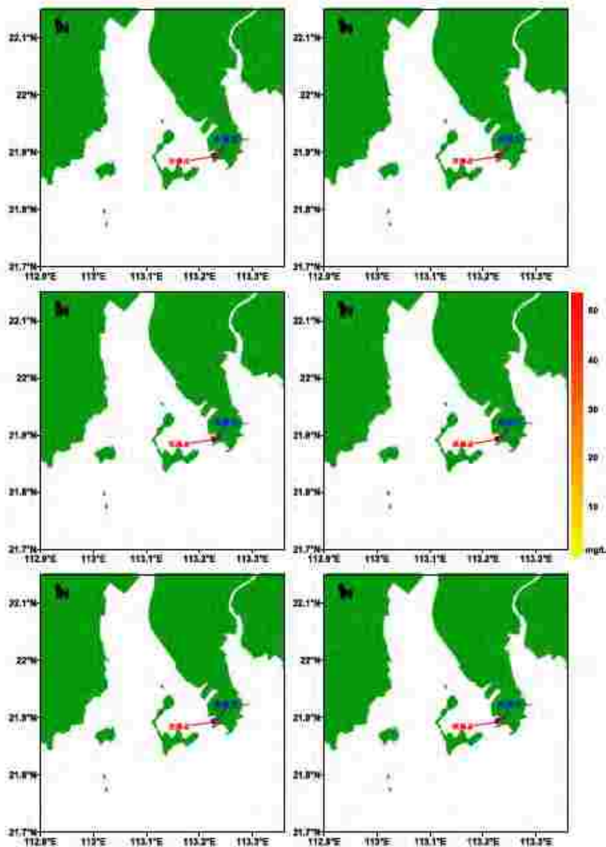
图9.3-8 冬季主导风落潮时码头前沿操作性溢漏事故硫酸漂移扩散预测结果 (从上至下、左至右为第1至第6小时; 包络线浓度为 0.20\mu\text{g/L} )
