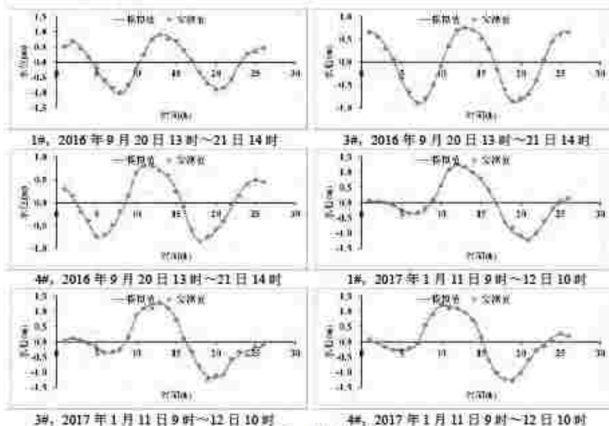
图 7.1-2 水位验证图
