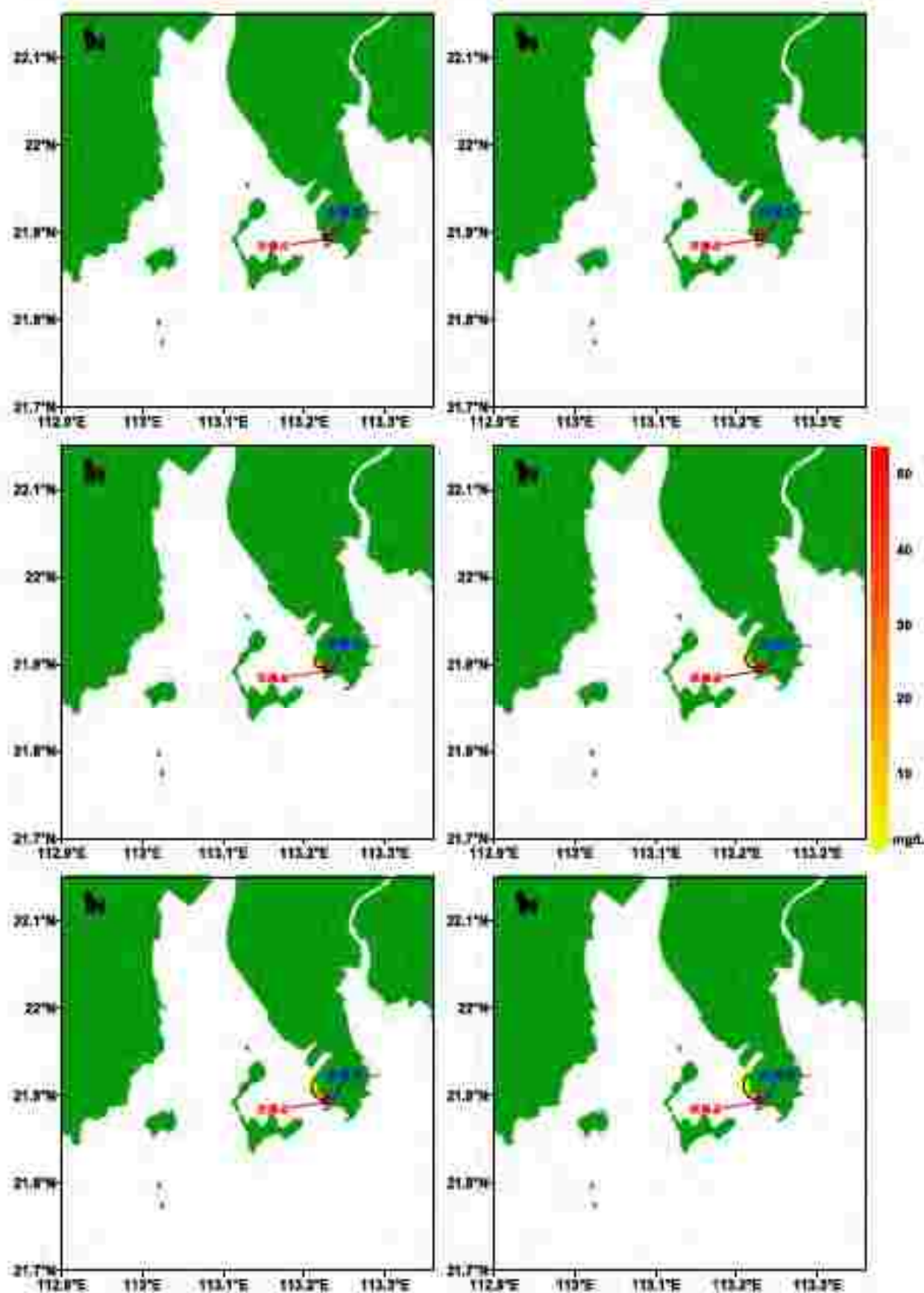
图9.3-7 冬季主导风涨潮时码头前沿操作性溢漏事故硫酸漂移扩散预测结果 (从上至下、左至右为第1至第6小时; 包络线浓度为 0.20\mu\text{g/L} )
