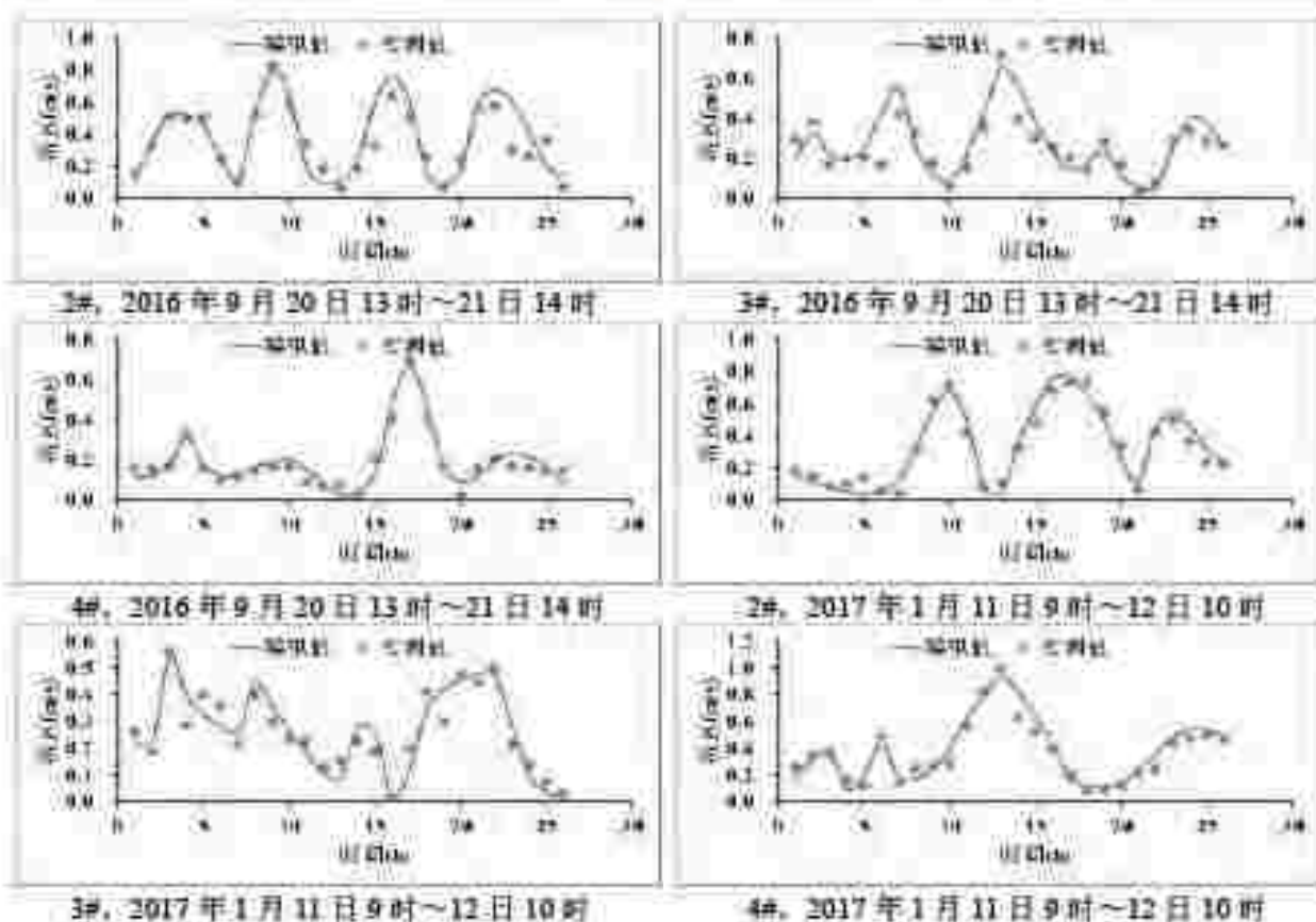
图 7.1-3 流速验证图
