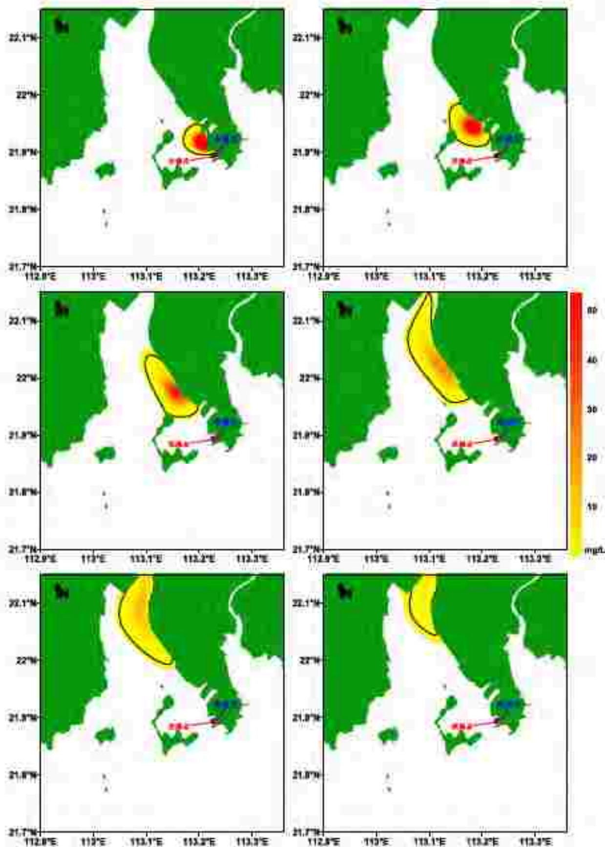
图9.3-11 不利风况涨潮时码头前沿操作性泄漏事故硫酸漂移扩散预测结果 (从上至下、左至右为第1至第6小时；包络线浓度为0.20ug/L)
