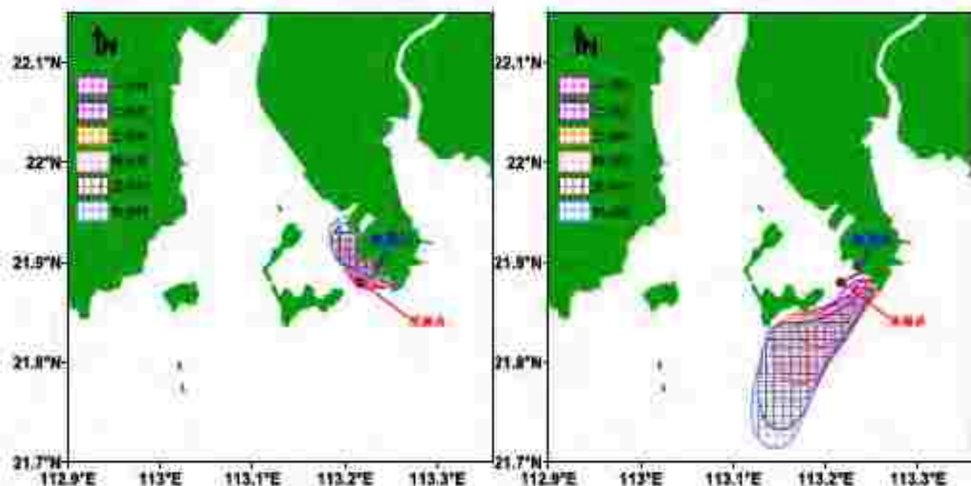
图9.3-13 海难性泄漏事故石油油膜漂移扩散预测结果
