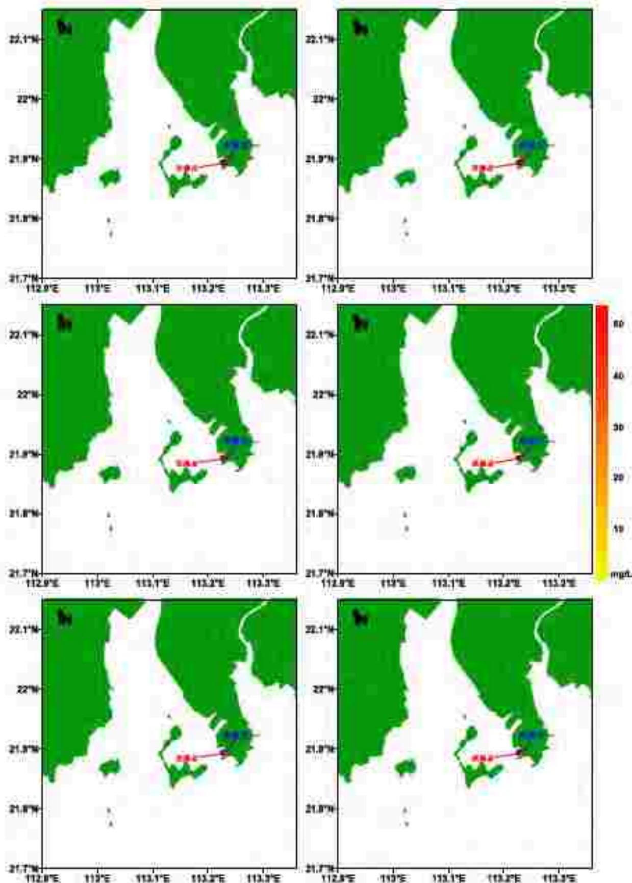
图9.3-10 夏季主导风落潮时码头前沿操作性泄漏事故硫酸漂移扩散预测结果 (从上至下、左至右为第1至第6小时; 包络线浓度为 0.20\mu\text{g/L} )
