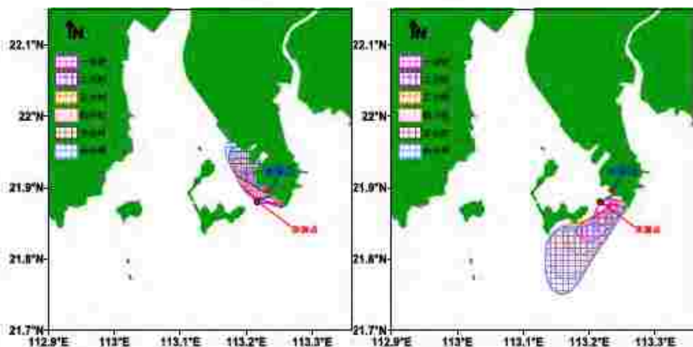
图9.3-14 海难性泄漏事故石油油膜漂移扩散预测结果
