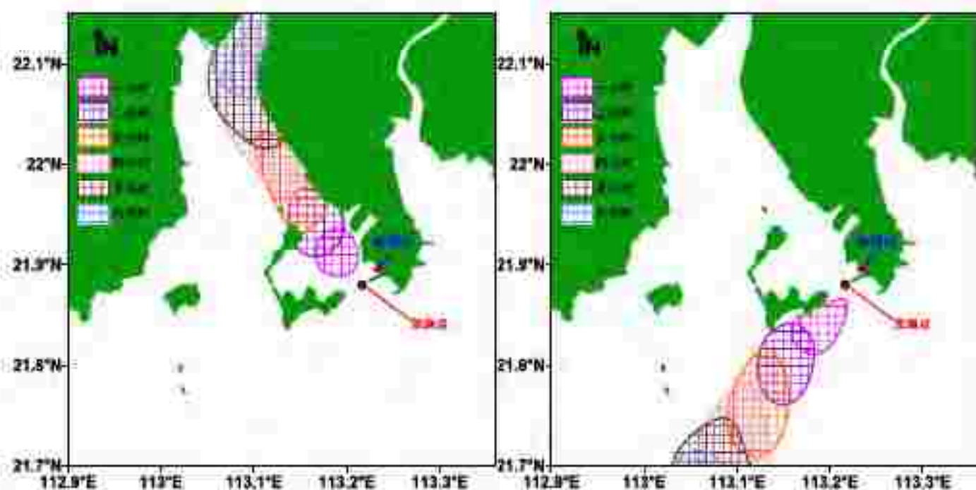
图9.3-18 海难性溢漏事故混合芳烃漂移扩散预测结果
