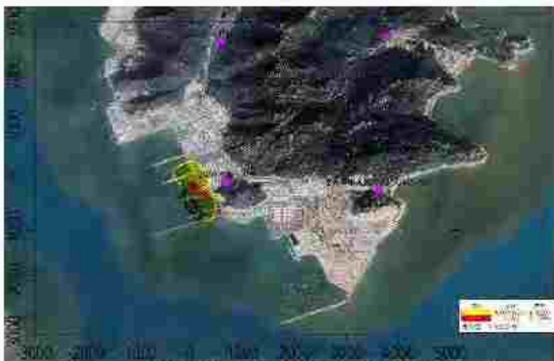
图 8.2-11 1#+3#泊位靠船时 SO 2 叠加现状浓度后年平均质量浓度分布图(μg/m 3 )
