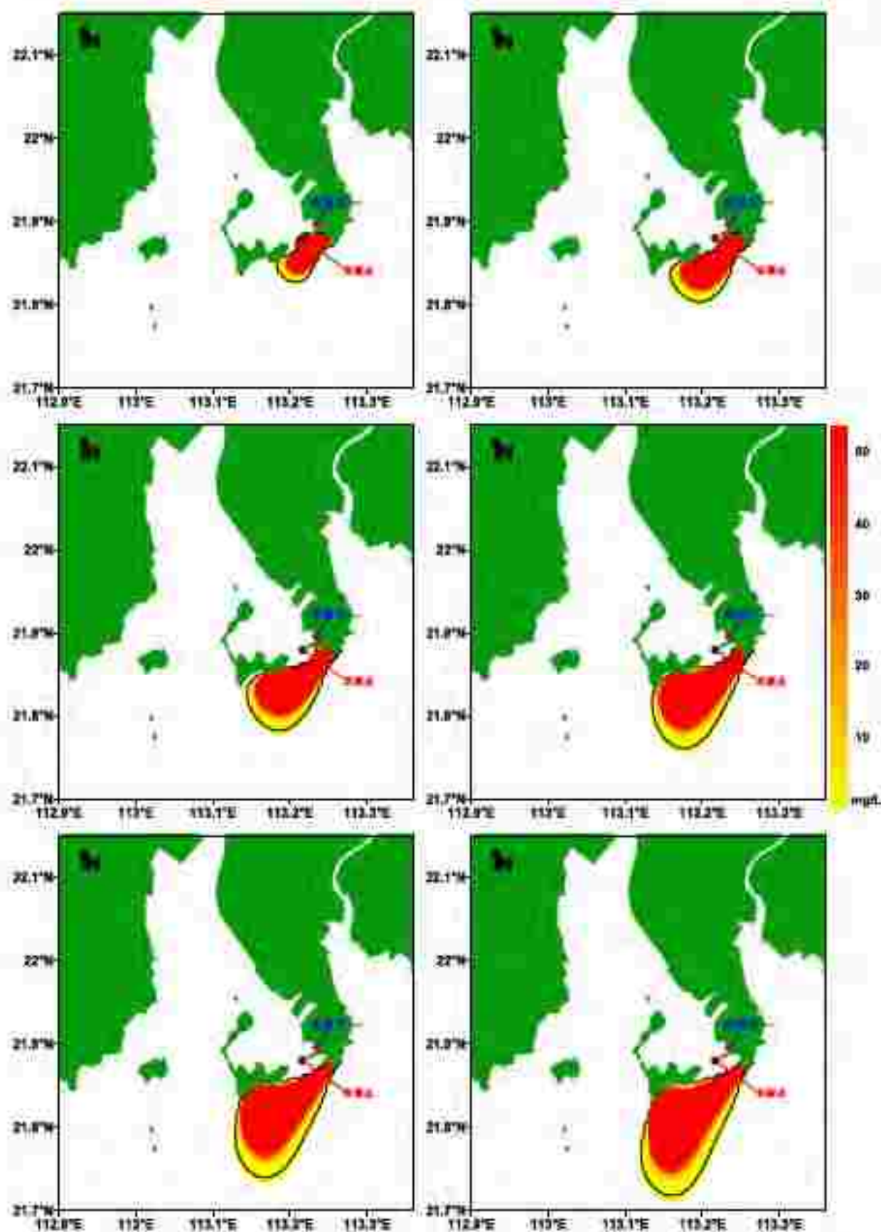
图9.3-22 夏季主导风落潮时码头前沿操作性泄漏事故硫酸漂移扩散预测结果 (从上至下、左至右为第1至第6小时; 包络线浓度为 0.20\mu\text{g/L} )
