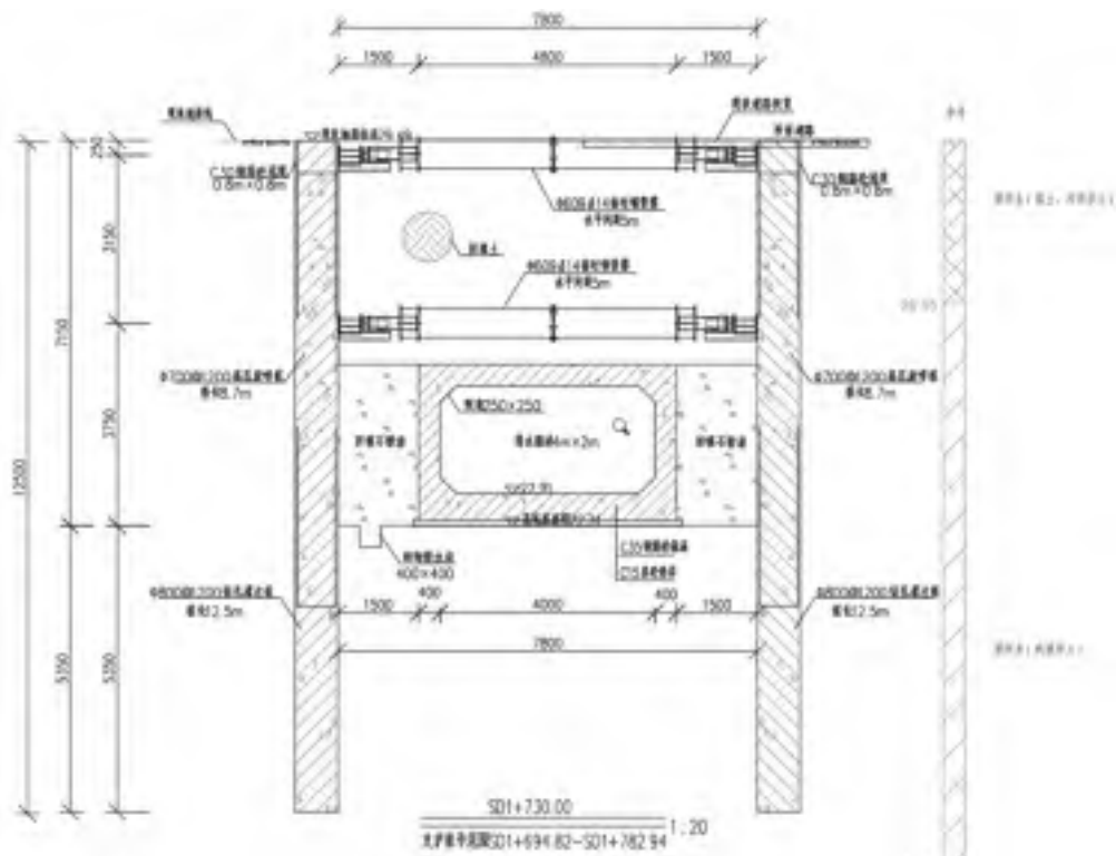
图 2.6-10 箱涵开挖支护典型断面
