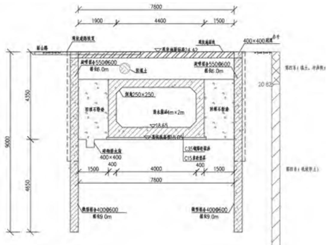
图 2.6-14 箱涵开挖支护典型断面
