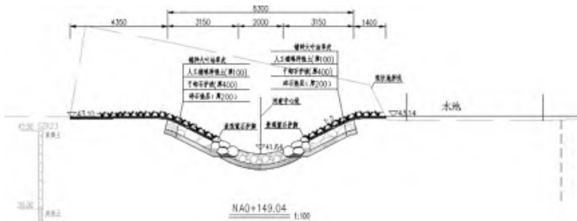
图 2.6-7 明渠典型横断面（六）
