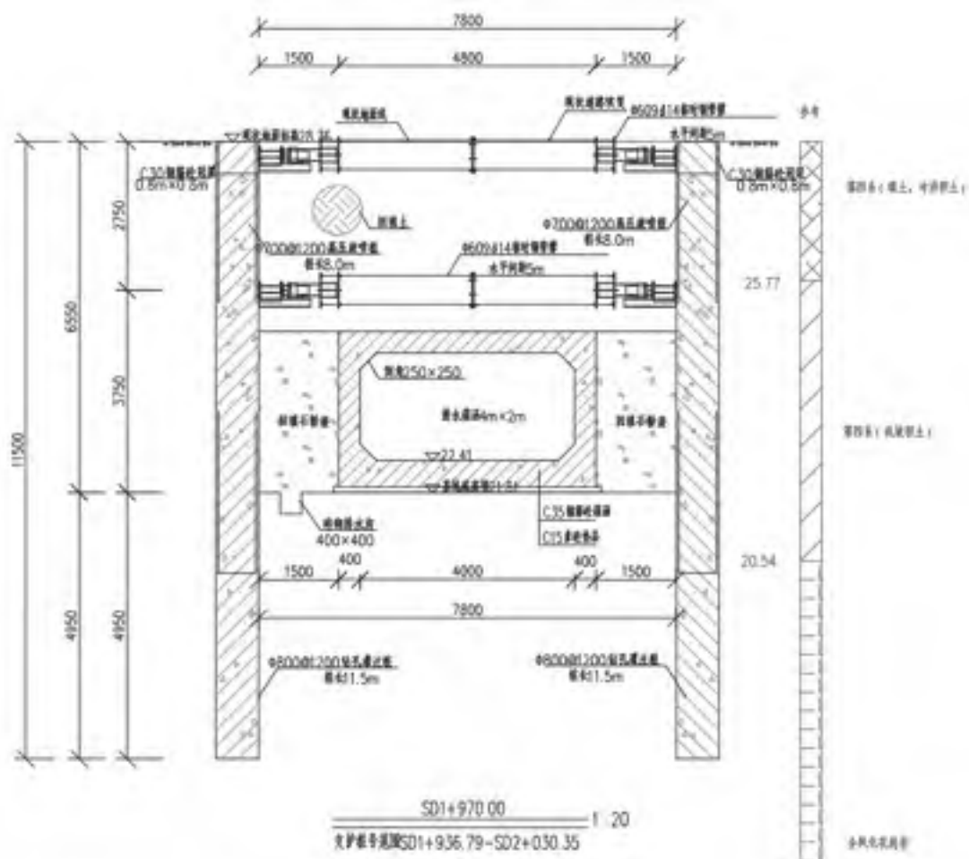
图 2.6-12 箱涵开挖支护典型断面
