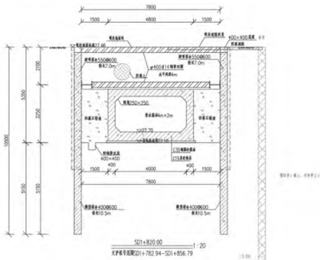
图 2.6-11 箱涵开挖支护典型断面
