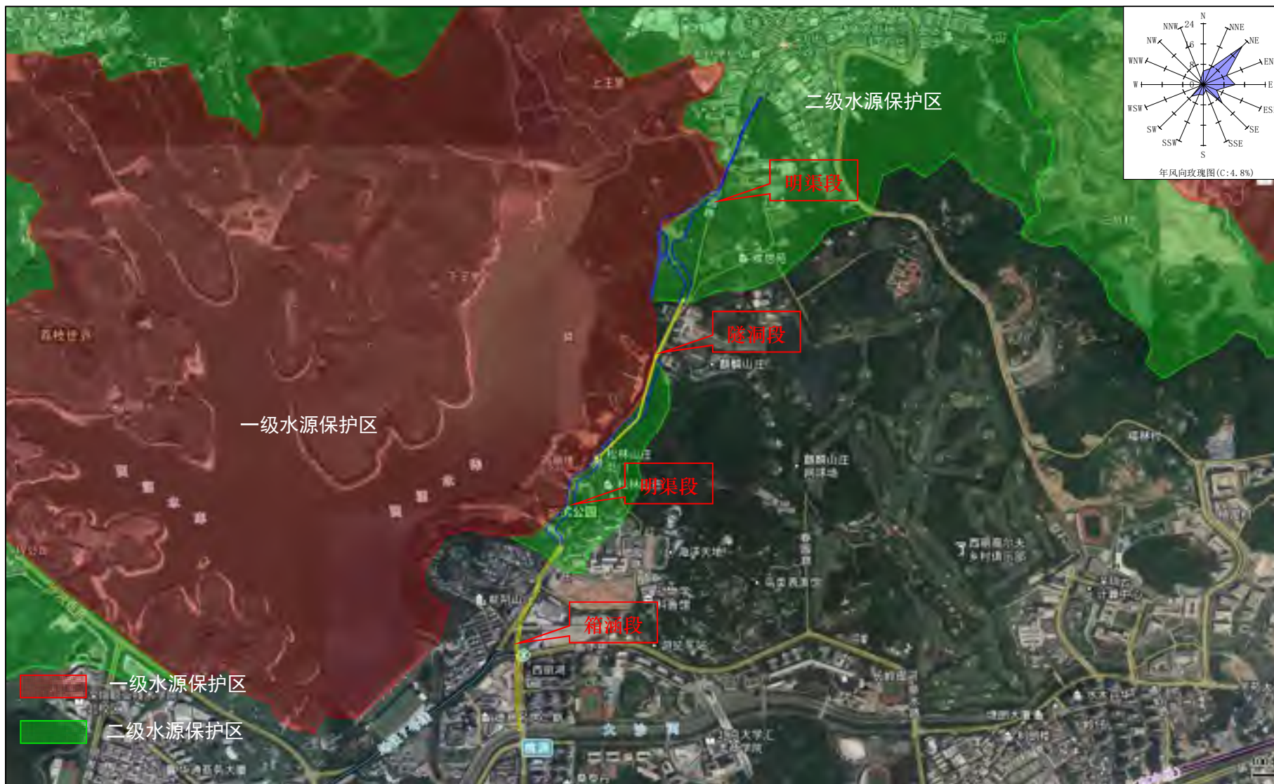
图 1.3-2 本工程与水源保护区的关系图
