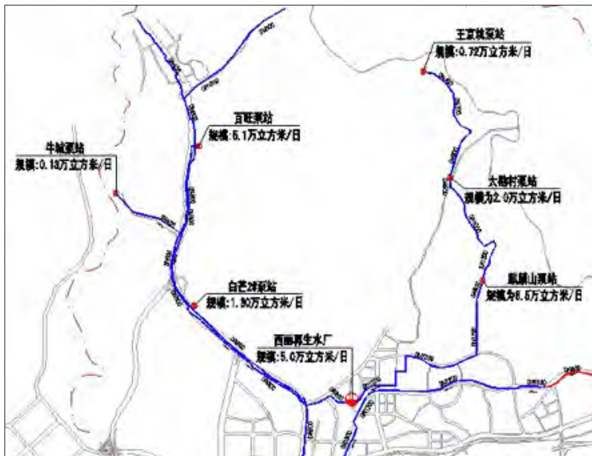
图 2.3-1 西丽水库环库截污干管系统示意图
