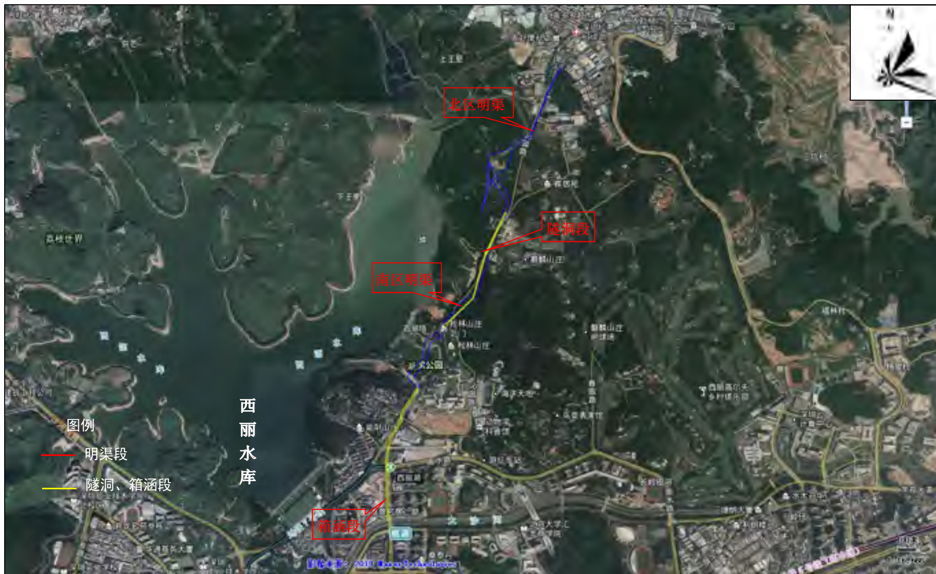
图 2.1-2 本工程的位置图
