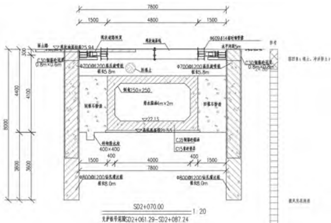
图 2.6-13 箱涵开挖支护典型断面
