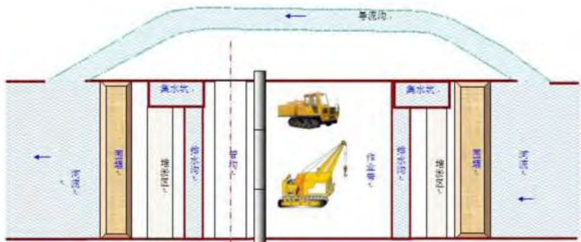
图 4.1-7 围堰导流开挖穿越河流
