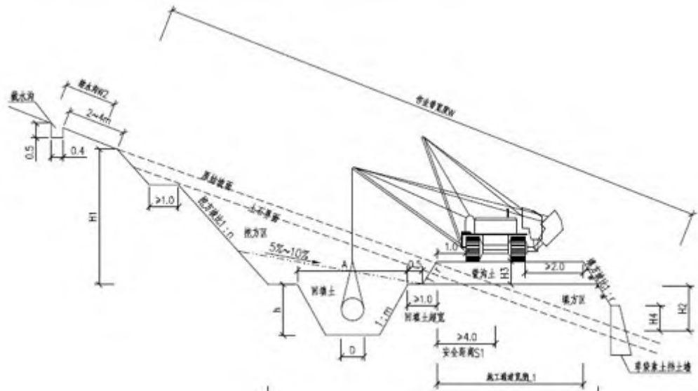
图 3.4-2 (B) 山地、丘陵段横坡敷设管道施工作业带示意图
