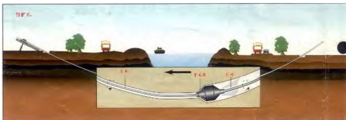
图 4.1-3 预扩孔示意
