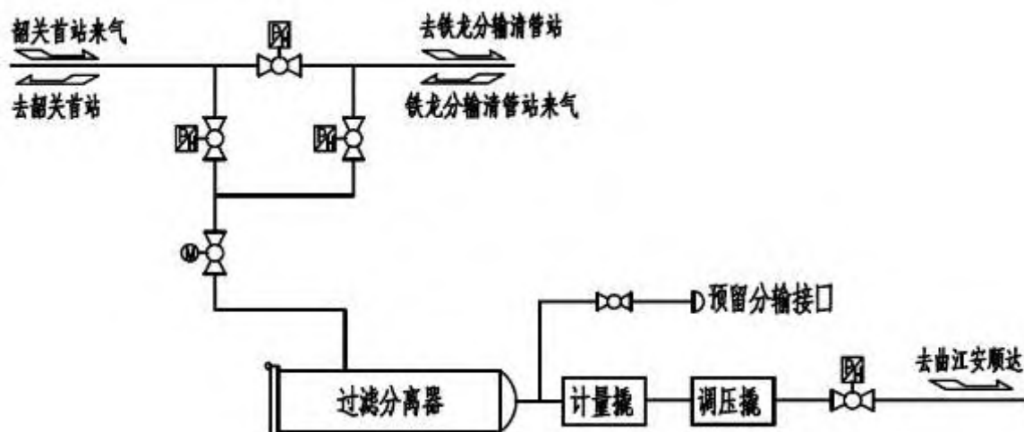
图 3.2.2-1 曲江分输站流程示意图
