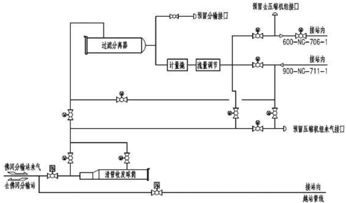
图 3.2.7-1 鳌头首站流程示意图
