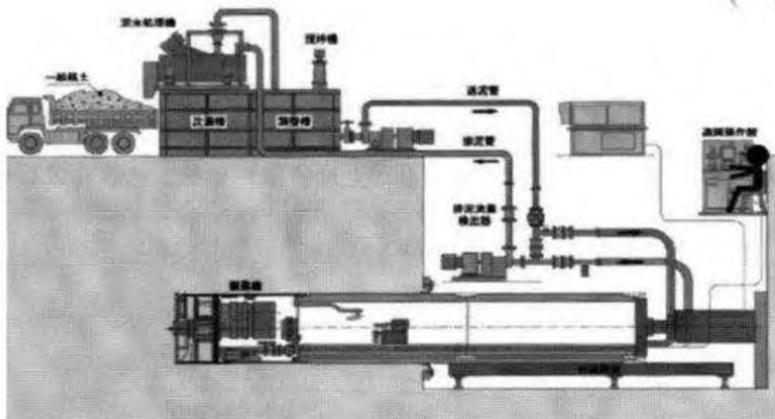
图 4.1-9 顶管穿越示意
