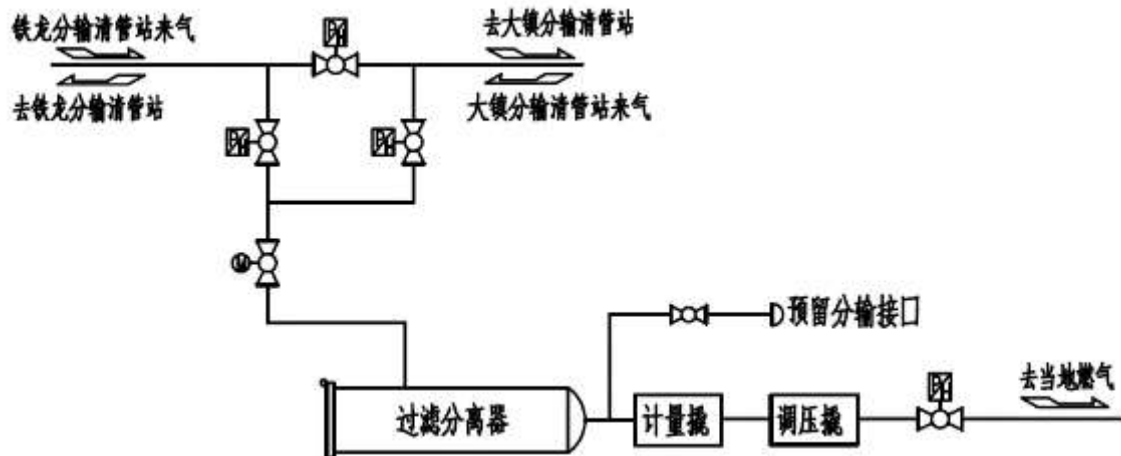
图 3.2.4-1 翁源分输站流程示意图
