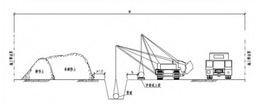
图 3.4-2 (A) 平地段管道施工作业带示意图
