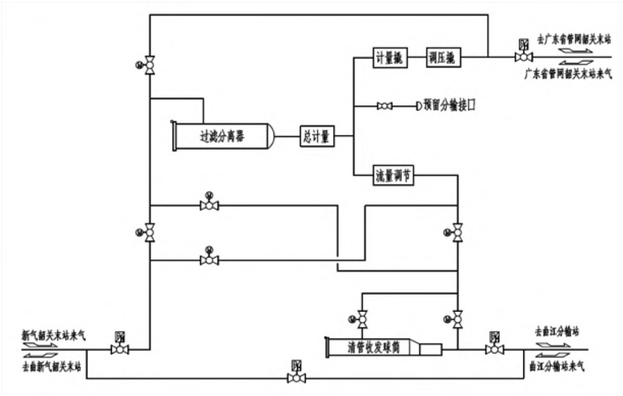
图 3.2.1-1 韶关首站流程示意图
