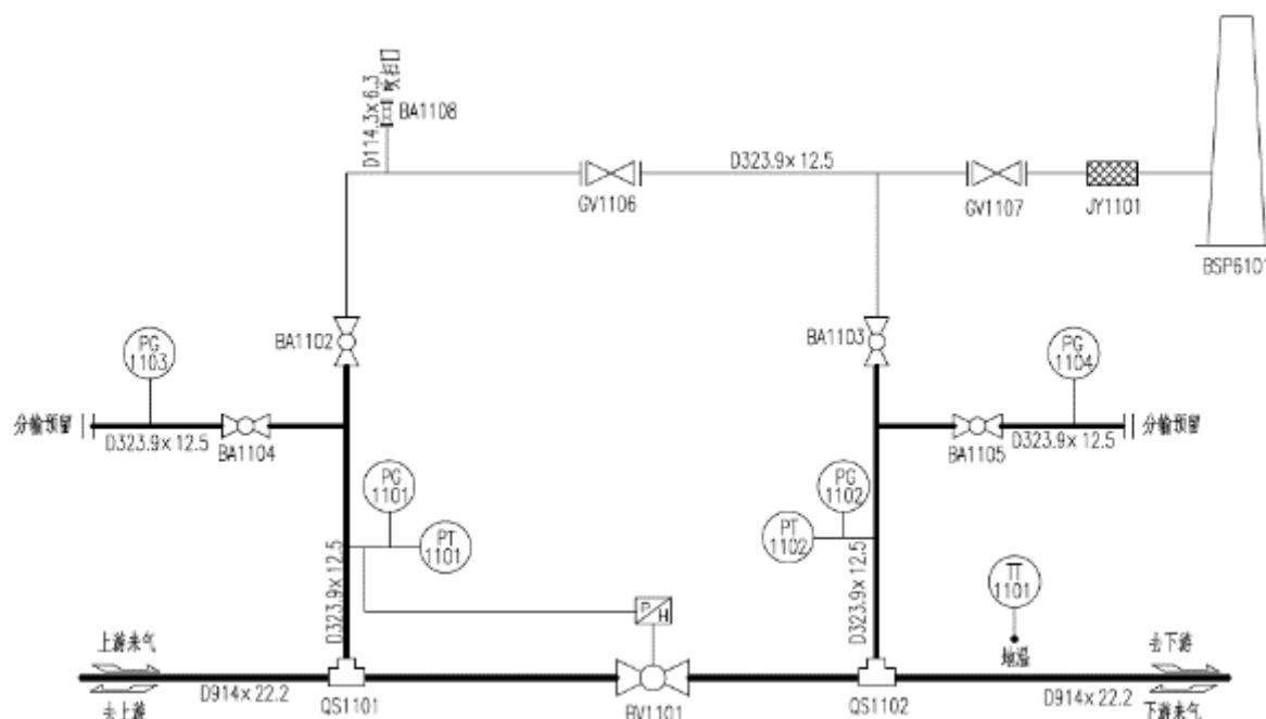
图 3.2.10-1 典型阀室流程示意图
