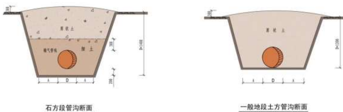
图 3.4-1 不同地段管沟断面示意图
