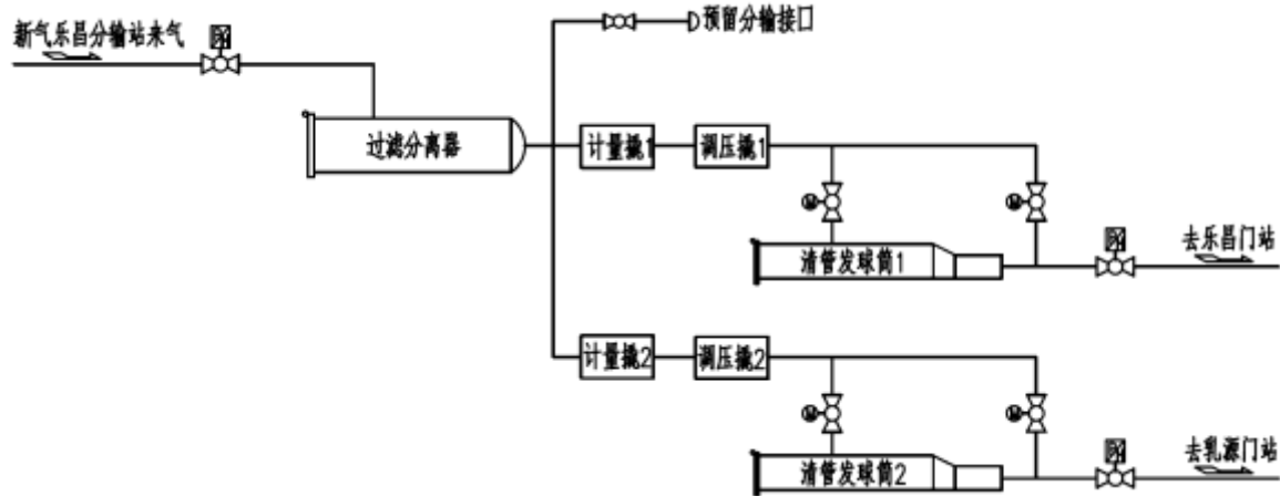
图 3.2.9-1 乐昌分输站流程示意图
