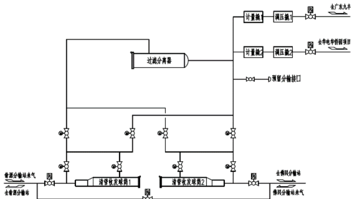
图 3.2.5-1 大镇分输清管站流程示意图
