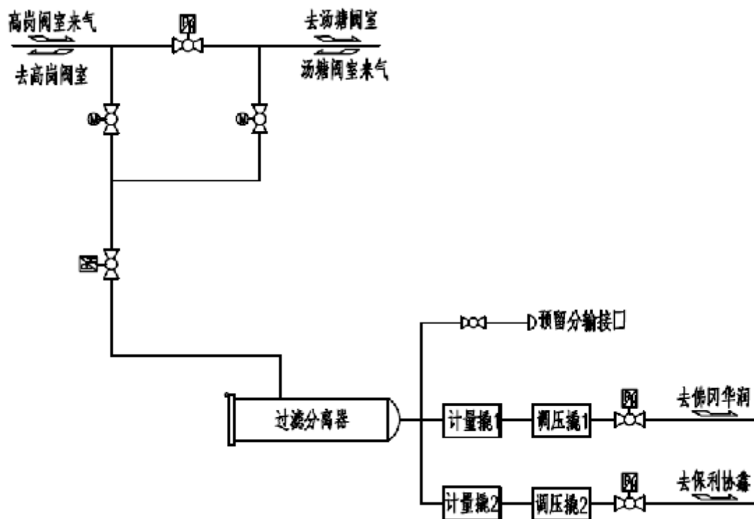
图 3.2.6-1 佛冈分输站流程示意图
