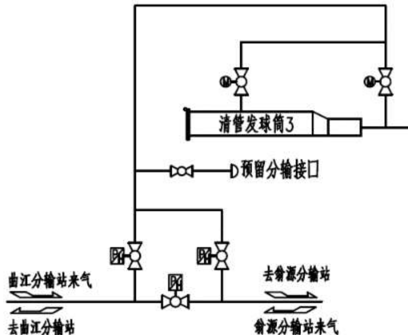
图 3.2.3-1 铁龙分输清管站流程示意图
