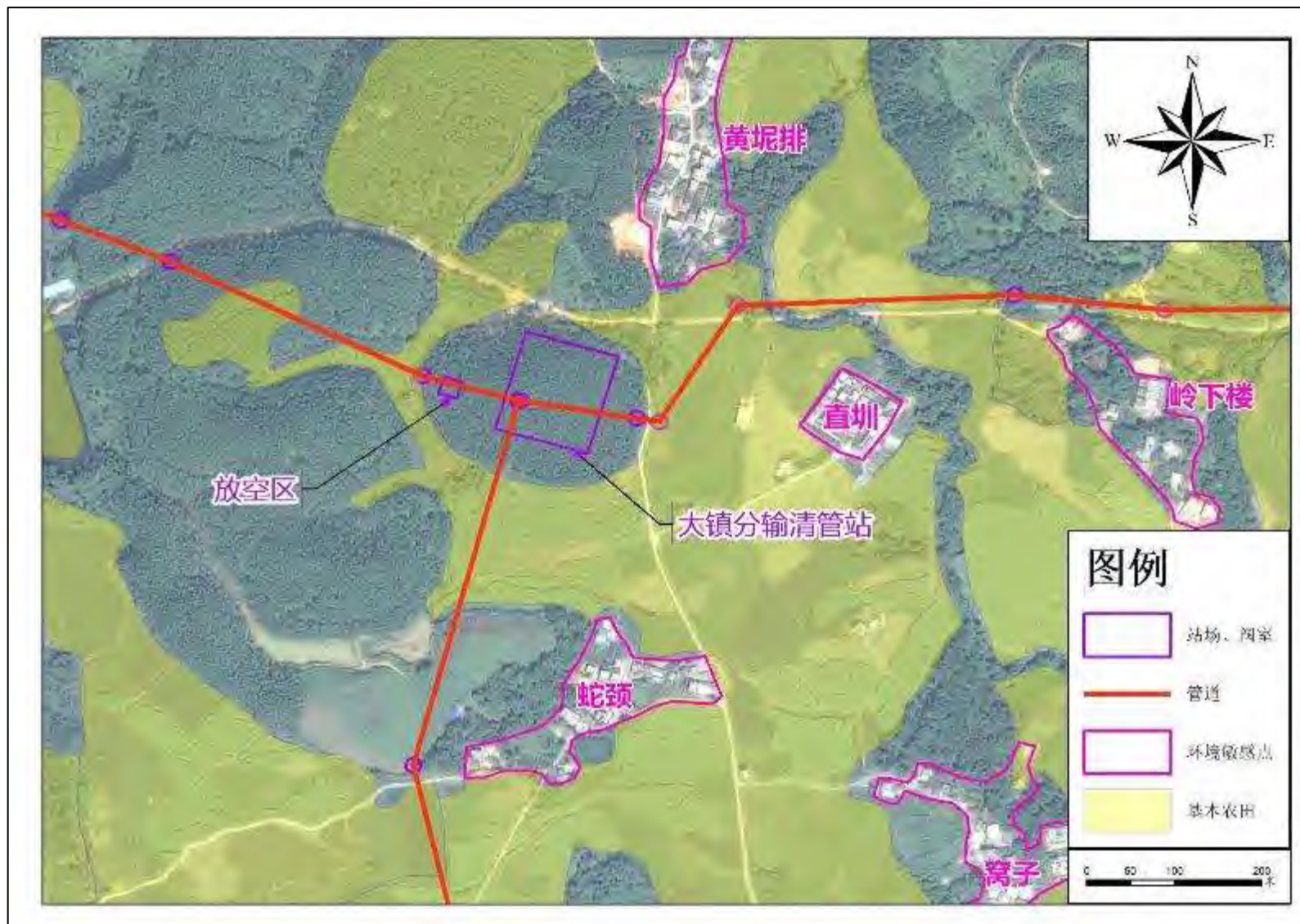
图 3.4-34 大镇分输清管站四至图
