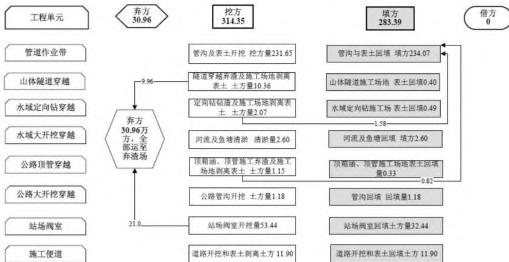
图 3.8-1 土石方量流向框图 (单位:万 m³)
