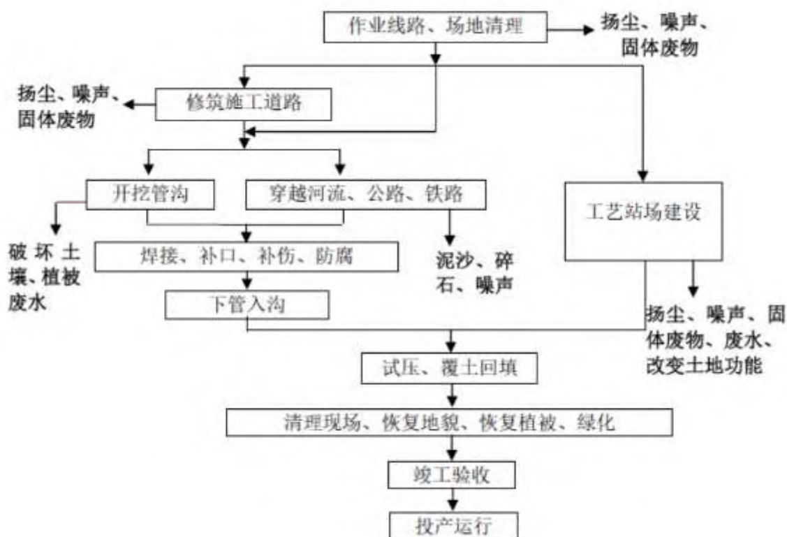
图 4.1-1 管道及站场施工流程及影响示意
