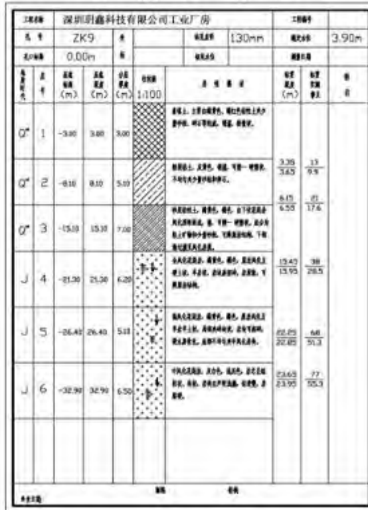
钻孔柱状图
