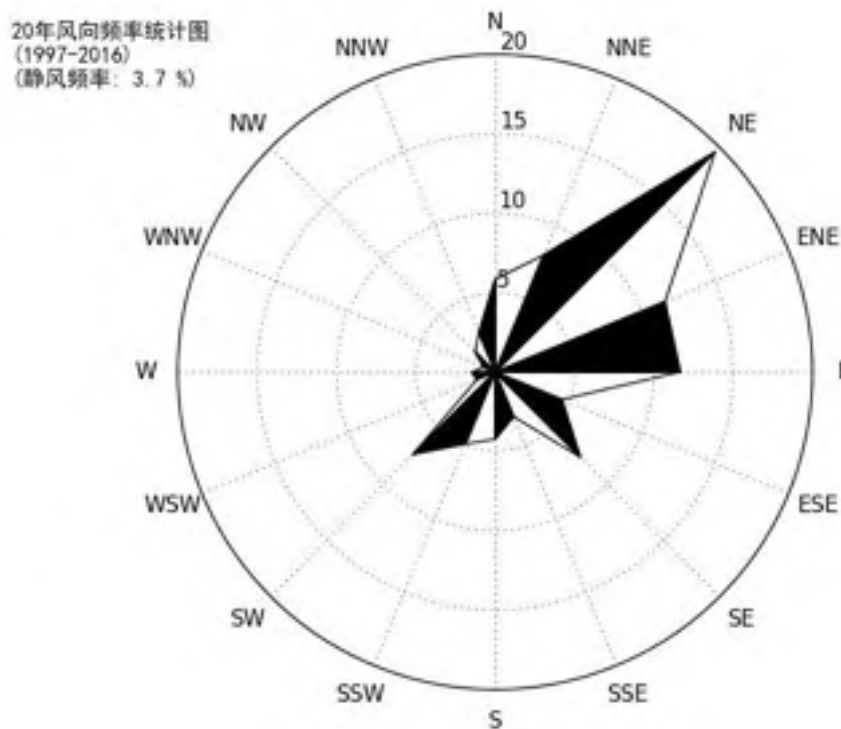
图5.1-1深圳市局大气成分站风向玫瑰图（静风频率 3.7%）（1997-2016年）
