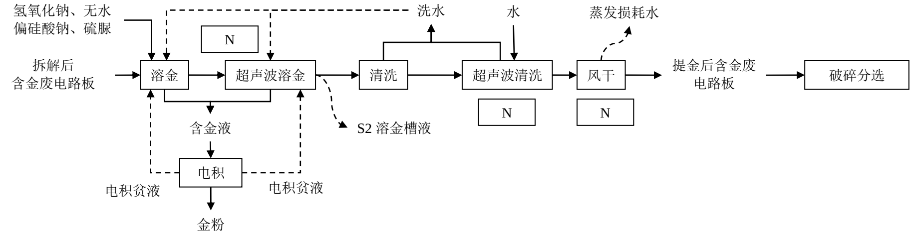
图 3.3-2 含金废电路板提金工序工艺流程及产污环节分析图
