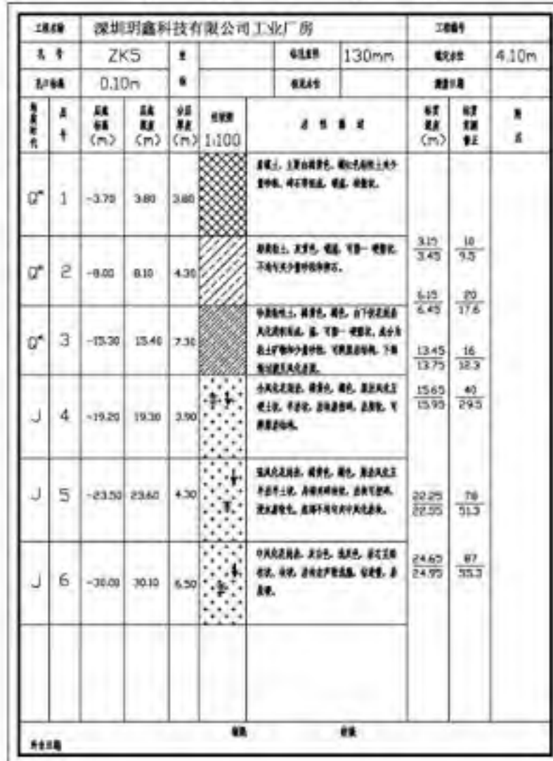
钻孔柱状图
