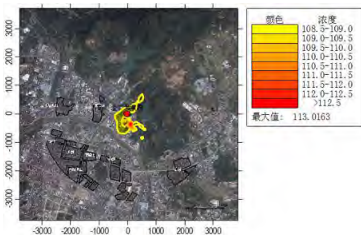
图 5.1-6 PM 10 叠加现状浓度后 95%保证率日均质量浓度分布图( \mu\text{g}/\text{m}^3 )
