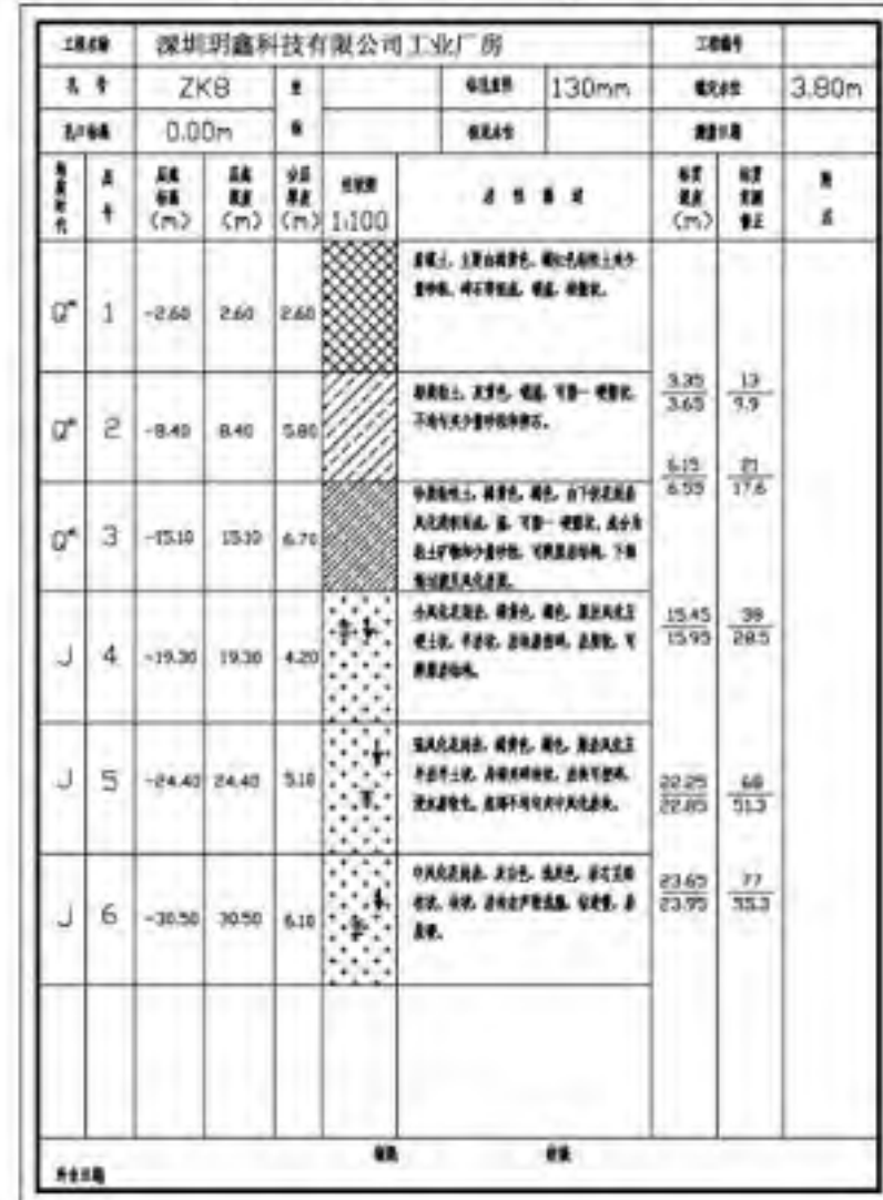
钻孔柱状图
