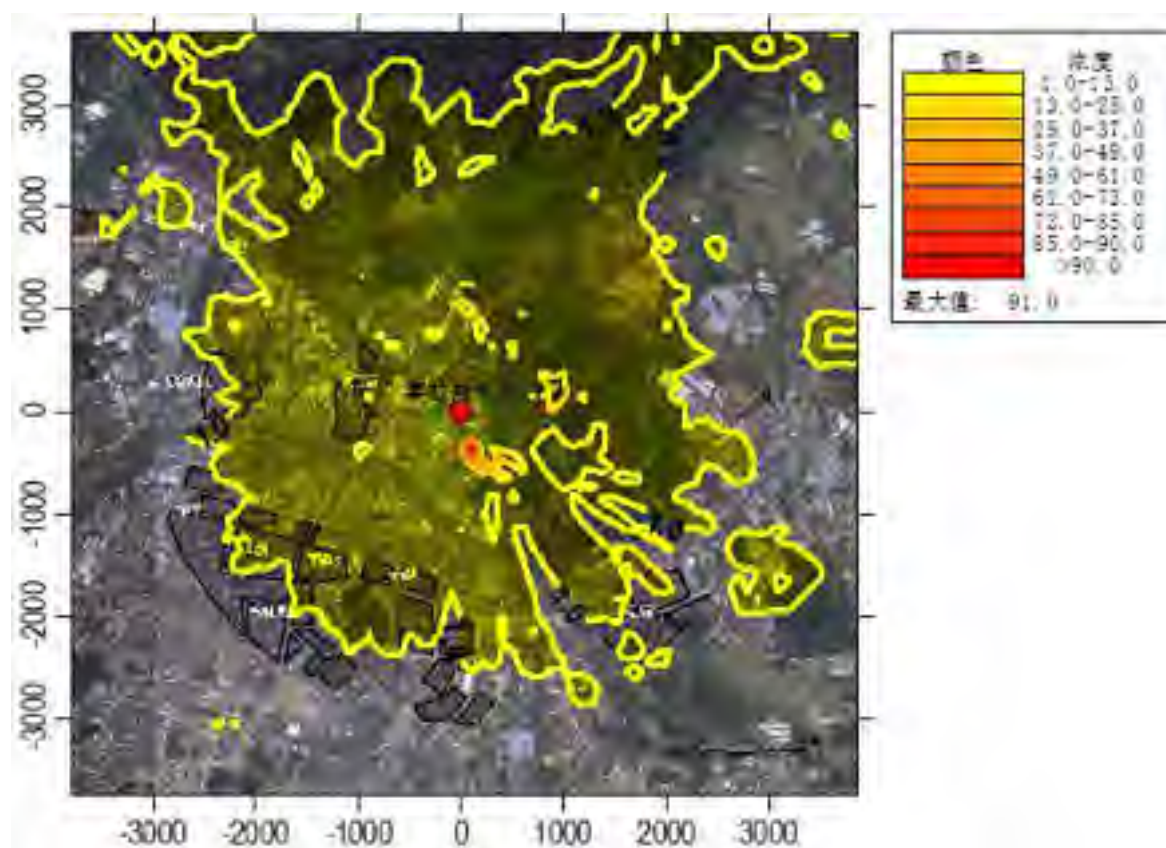
图 5.1-12 非正常排放下，非甲烷总烃小时平均浓度贡献值分布图(µg/m 3 )
