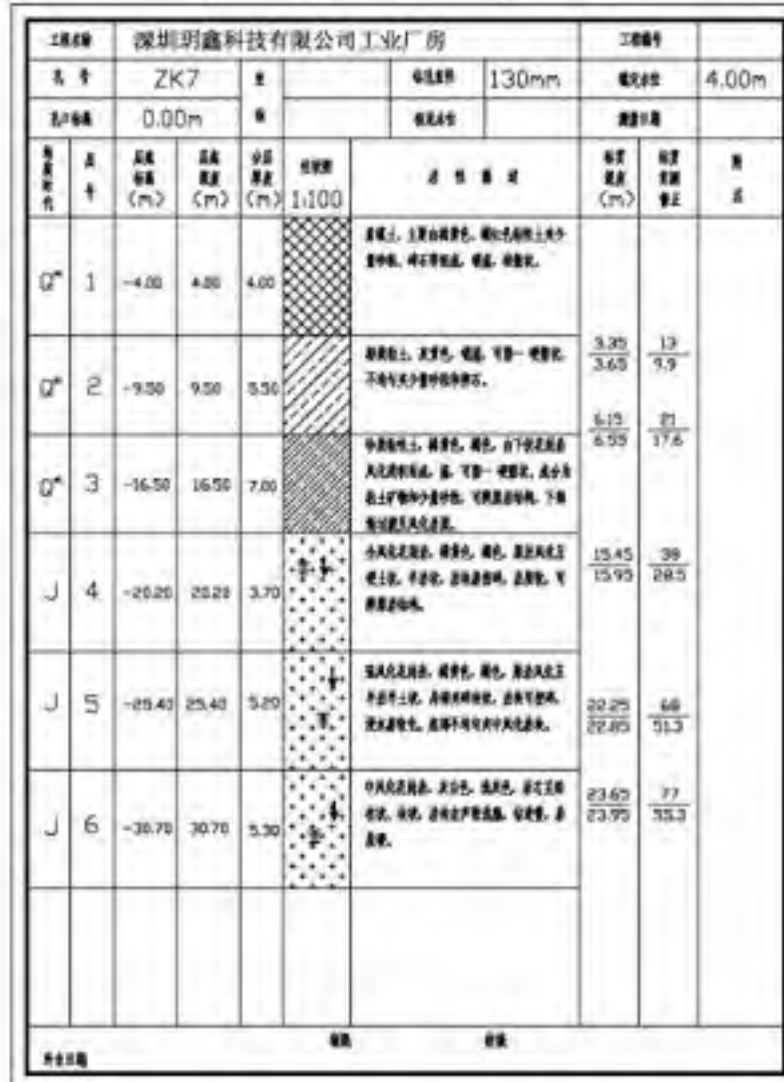
钻孔柱状图
