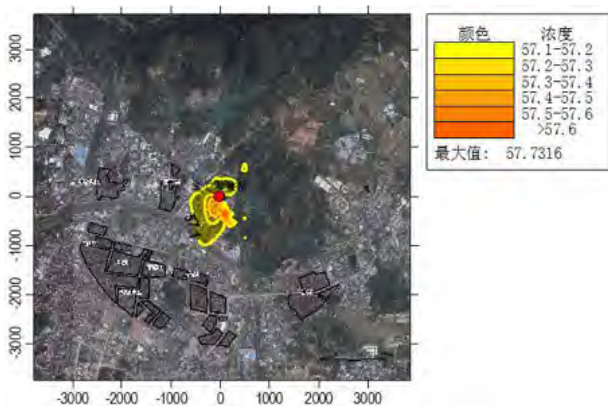
图 5.1-7 PM 10 叠加现状浓度后年平均质量浓度分布图( \mu\text{g}/\text{m}^3 )
